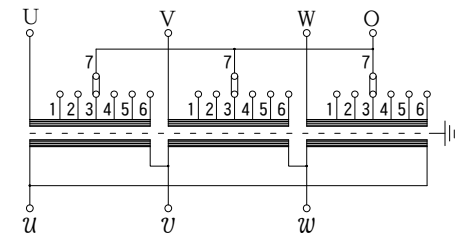
結線図
