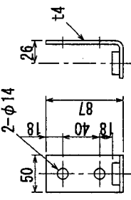
二次端子詳細図
