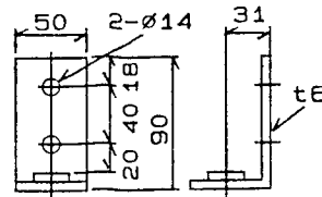
一次端子詳細図
