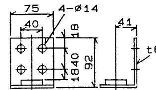
二次端子詳細図
