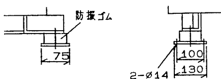
防振ゴム(別送)詳細図
