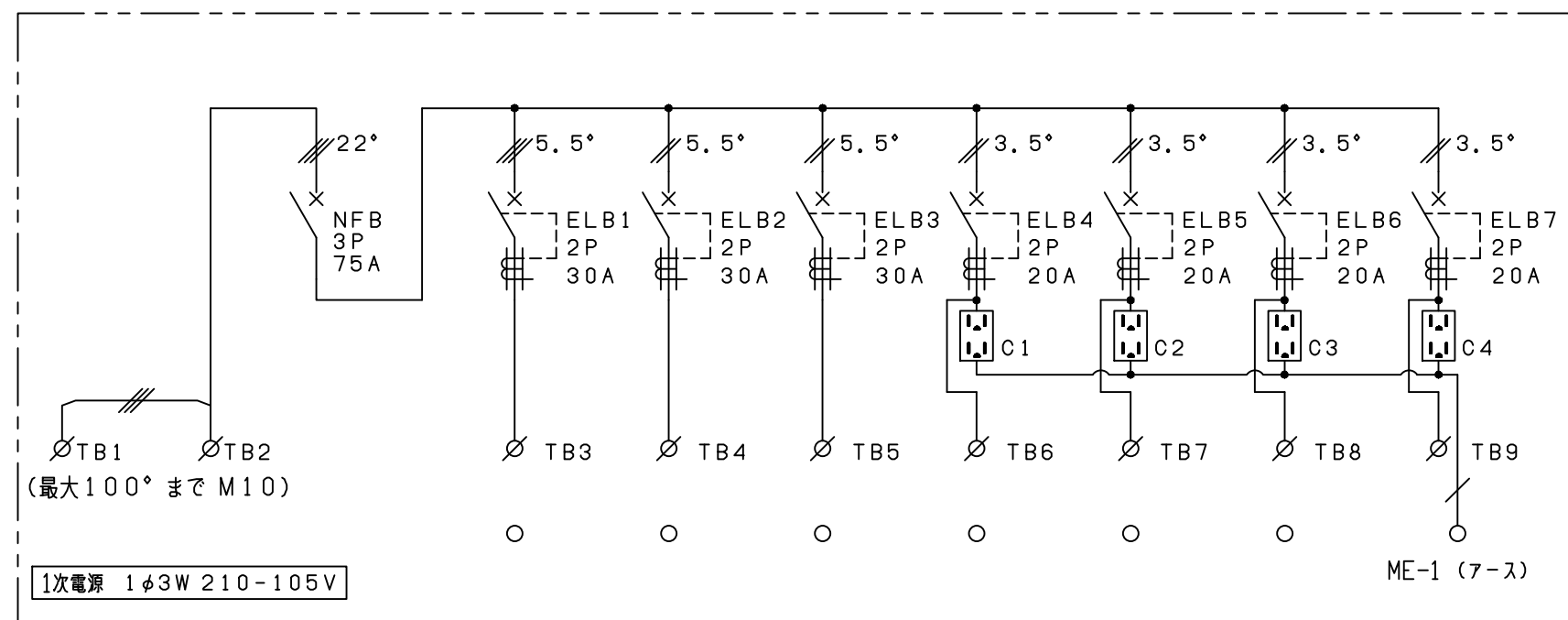
結線図
