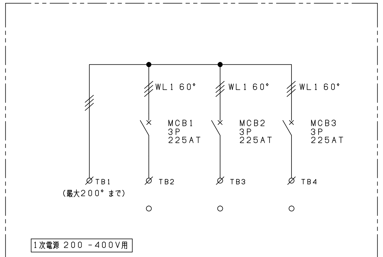
結線図
