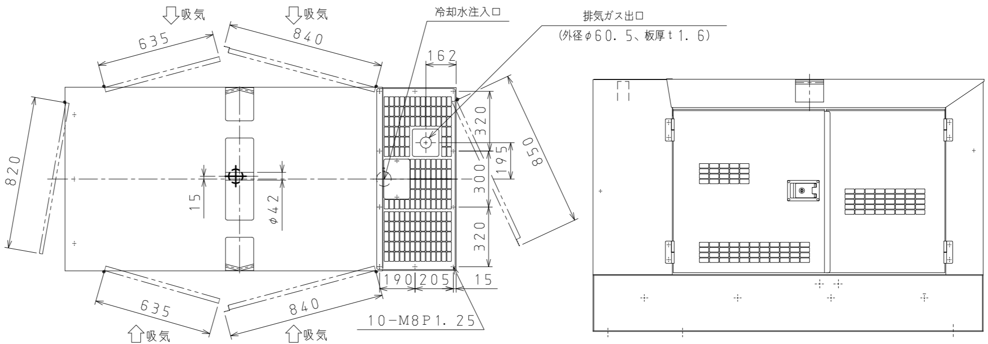
A 矢視図
