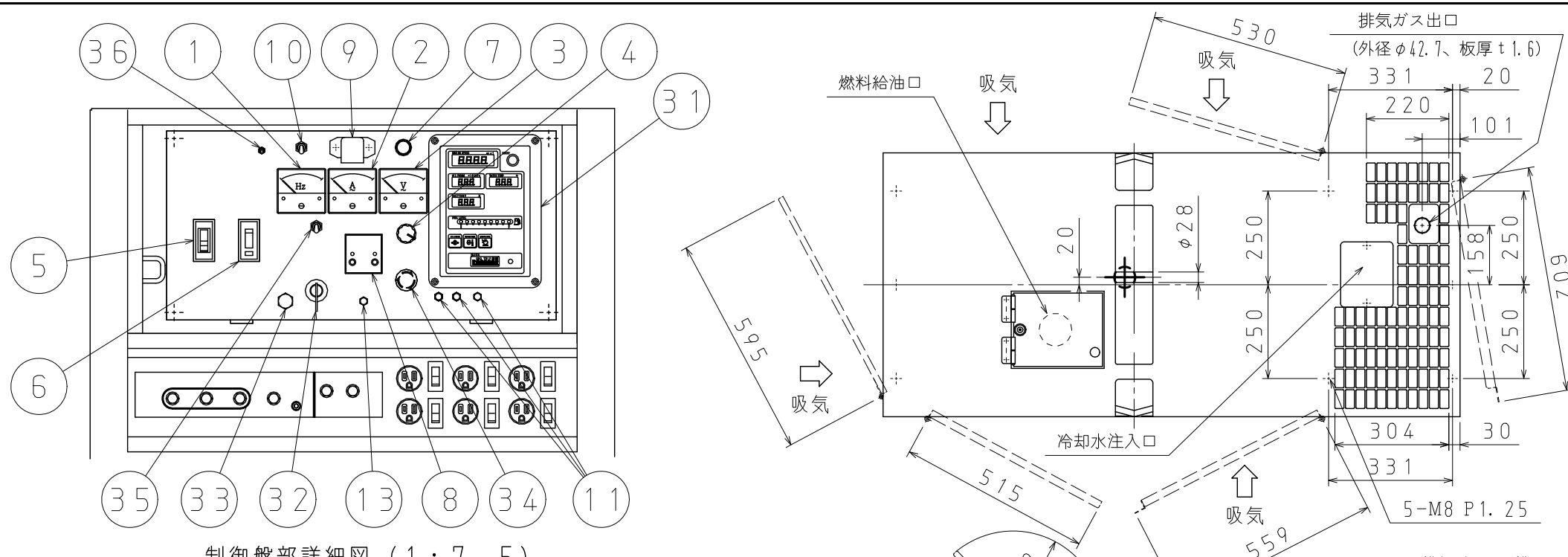
制御盤部詳細図 (1:7.5)
