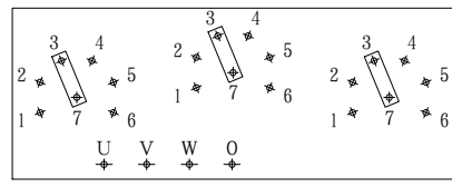
SEC 2.3t 電圧切替端子板
