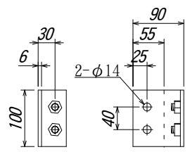
1次、2次端子
