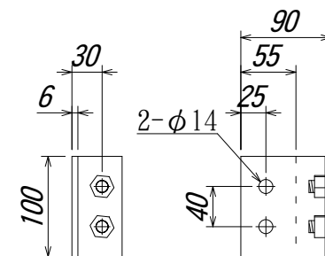
1 次, 2 次端子
