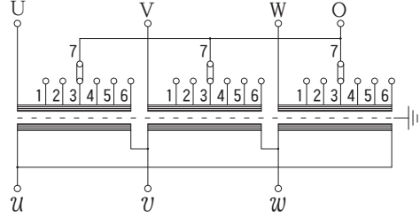
結線図
