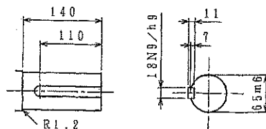
軸端詳細
