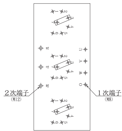
電圧切替端子板詳細
