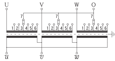
結線図
