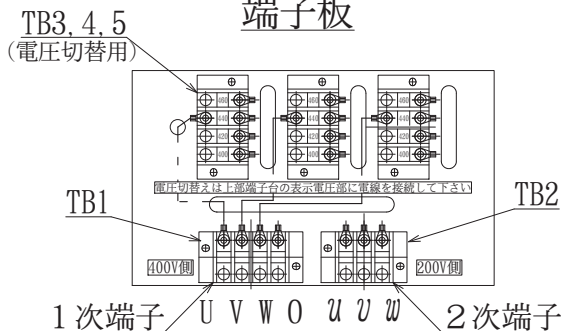
端子板
