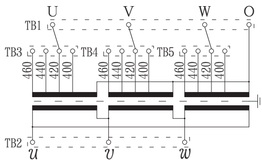
端子板
