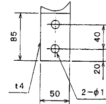
(二次端子詳細)
