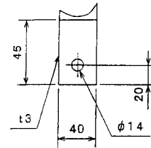
(一次端子詳細)
