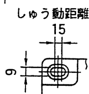
取付足を上側より見て
