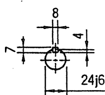
断面 A A
