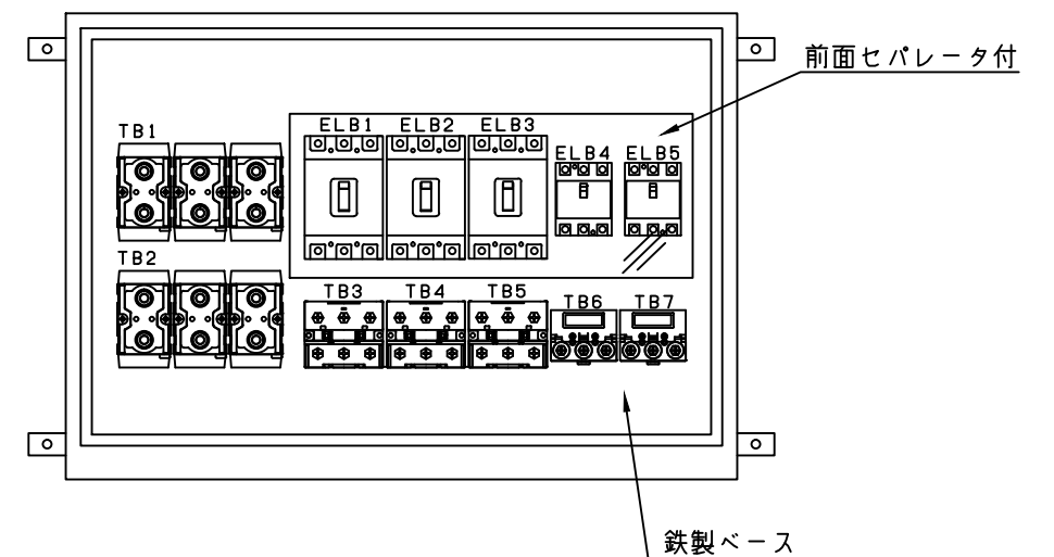
配置図
