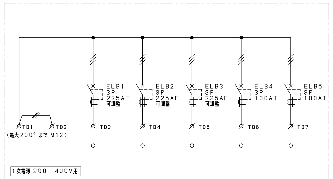
結線図
