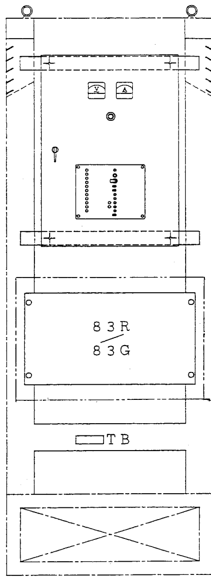
正面図 TB ATL15L 10P
