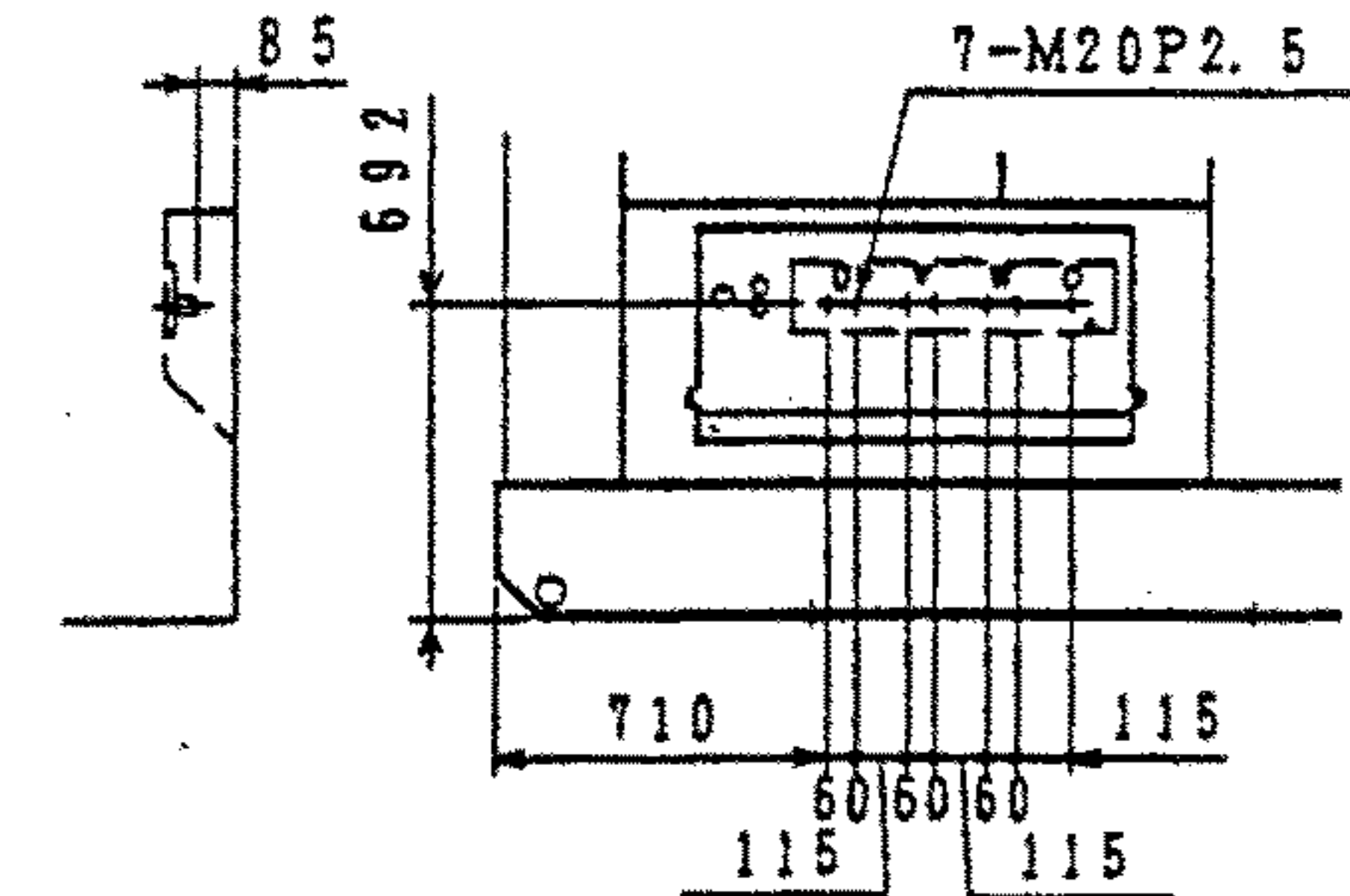
出力端子部詳細図
